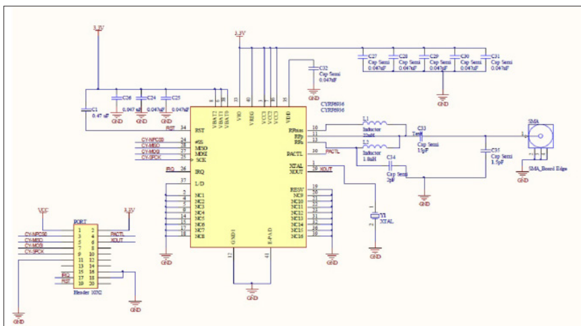
تصویر ۱۲- مدار فرستنده و گیرنده.
