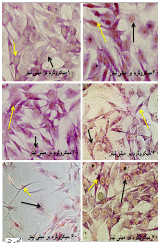
تصویر ۴- سلول‌های شبه عصبی القاء شده با عصاره Zingiber در غلظت‌های ۱۰، ۲۰، ۳۰، ۴۰، ۶۰ و ۷۰ میکروگرم بر میلی‌لیتر و به مدت ۲۴ ساعت.
