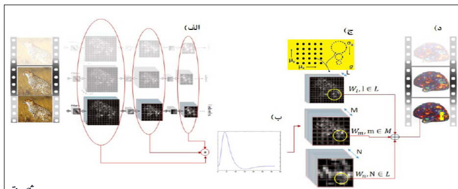
تصویر ۳- ساختار کلی مدل رمزگذاری با مفهوم میدان تأثیر. الف) نقشه‌های ویژگی با استفاده از شبکه کانولوشنی برای هر فریم ویدیو استخراج می‌گردد. ب) نقشه‌های استخراج شده با تابع همودینامیک کانالو می‌شود. ج) یک مجموعه از سایز و مکان میدان ادغام در نظر گرفته می‌شود. د) خروجی ناشی از اعمال میدان ادغام ویژگی بر روی نقشه‌های ویژگی را وزن‌دار کرده که این وزن‌ها از طریق گرادیان کاهشی بهینه می‌گردند.
