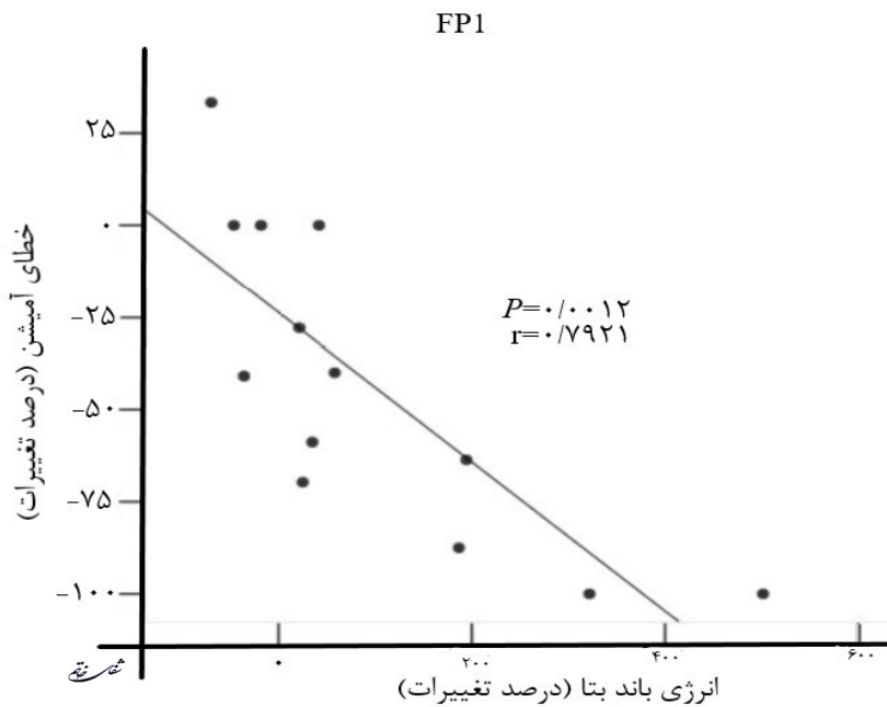
تصویر ۶- همبستگی بین درصد تغییرات انرژی بتا و درصد تغییرات خطای آمیشن در تحریک شنیداری هدف در کانال FP1
