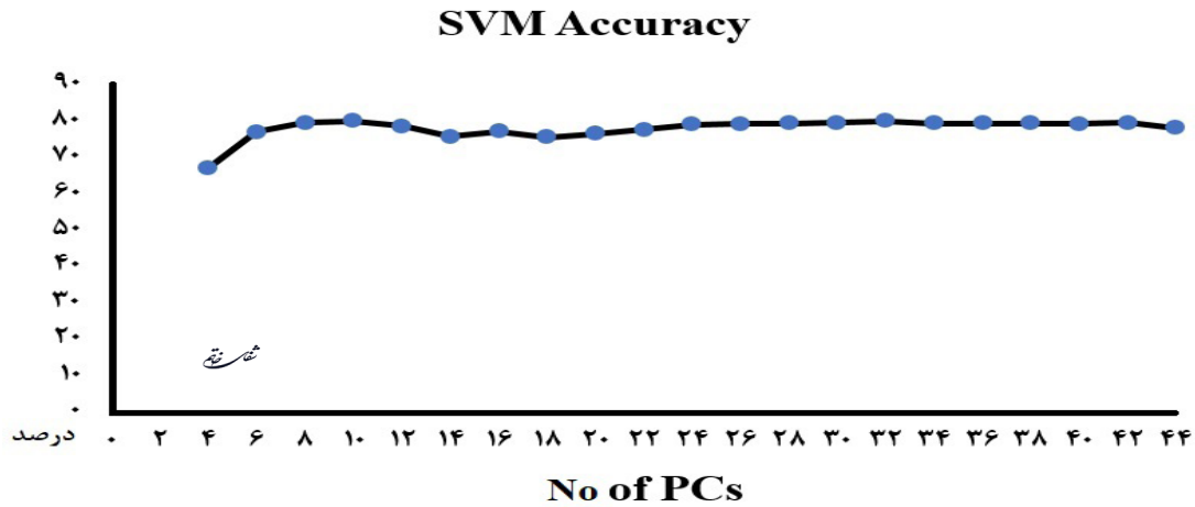
تصویر ۴- اثر اعمال الگوریتم PCA روی پارامتر دقت الگوریتم SVM
