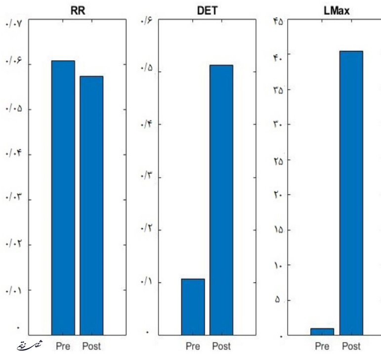
نمودار ۲- ویژگی‌های RQA سیگنال EEG در قبل و بعد از tDCS در داده‌های چشم باز
