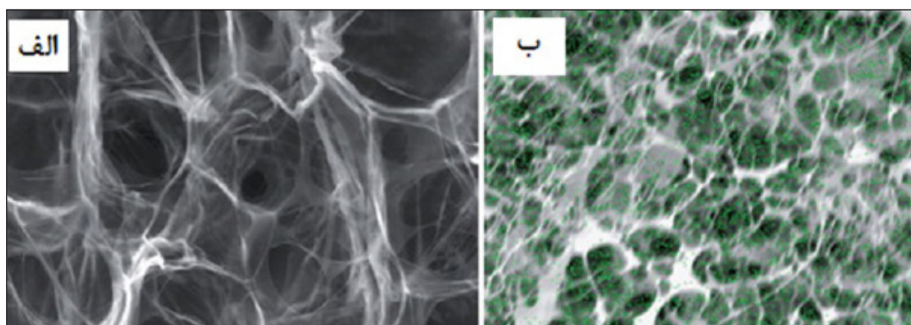
تصویر ۱- مقایسه تصاویر میکروسکوپ الکترونی اسکینینگ از داربست‌های کلاژنی (الف) و داربست کلاژنی/اسید هیالورونیک (ب).
