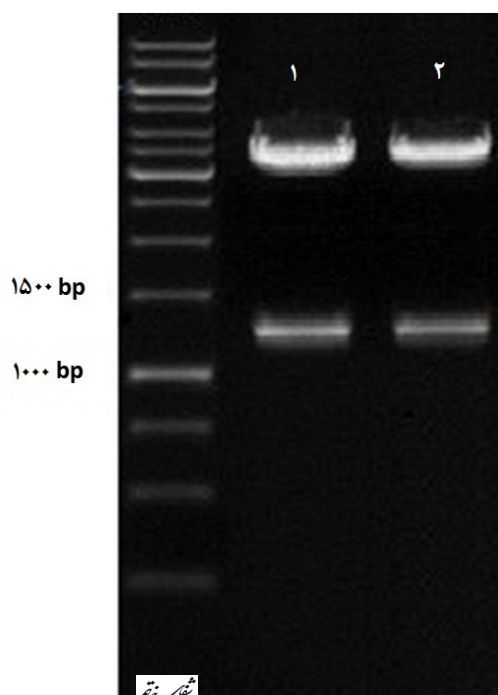
تصویر ۲- الکتروفورز پلاسمید ساب کلون شده pSecTag2-NGF به همراه پلاسمید pSecTag2. ستون سمت چپ (۱) GeneRuler DNA Ladder Mix (پلاسمید pSecTag2/Hygro با وزن حدود ۵۷۰۰ bp) (۲) پلاسمید ساب کلون شده pSecTag2-NGF با وزن حدود ۷۰۰۰ bp. پلاسمید ساب کلون شده به اندازه وزن ژن NGF افزایش وزن نشان می‌دهد.
