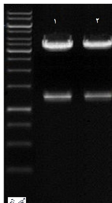
تصویر ۱- الکتروفورز پلاسمید حامل، بعد از مرحله هضم آنزیمی. ستون سمت چپ (GeneRuler 1 kb DNA Ladder) (۱ و ۲) پلاسمید pCMV-SPORT6 هضم آنزیمی شده و باند مربوط به NGF از آن جدا شده است.
