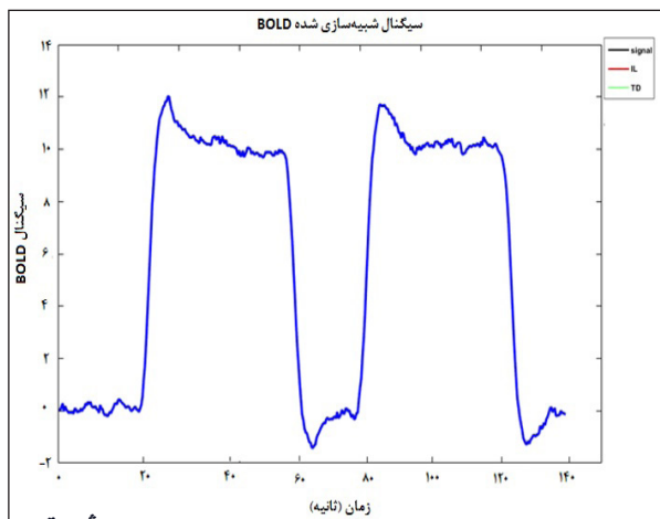
تصویر ۱- سیگنال شبیه‌سازی شده در طراحی بلوکی در نرم‌افزار متلب، TR=3 ثانیه، زمان‌های شروع تحریک ۶۰ و ۲۴۰ ثانیه، مدت هر تحریک ۱۲۰ ثانیه، طول بلوک ۴۲۰ ثانیه.
