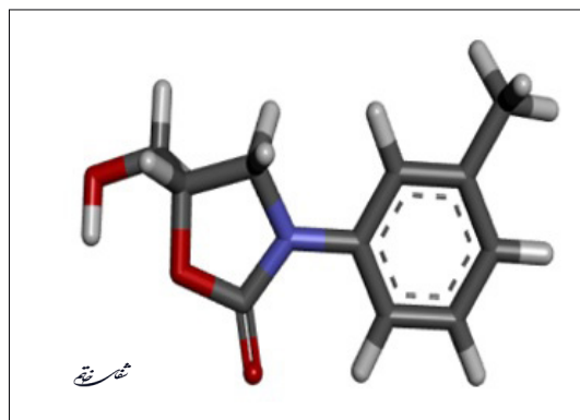
تصویر ۲- ساختار ترکیب مهارکننده تولوکسان که به عنوان ترکیب مهار رهر جهت فارماکوفور و جستجوی مجازی برای به دست آوردن لیگندهای مهار جدید مهارکننده آنزیم مونوآمینواکسیداز A- استفاده گردید.
