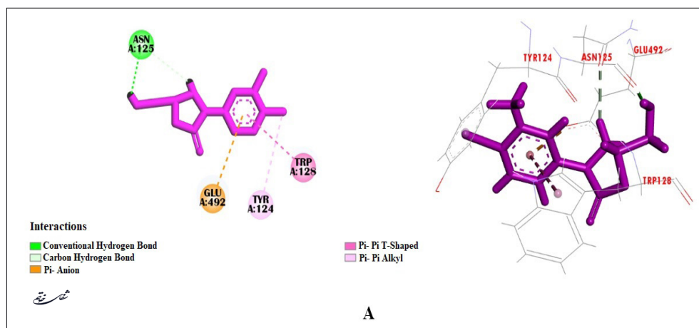
تصویر ۶- تصویر برهمکنش لیگاندهای به دست آمده با آنزیم مونوآمین اکسیداز-A با استفاده از نرم‌افزار دیسکوری استودیو. A (لیگاند ۴۶) و B (لیگاند ۴۸) و C (لیگاند ۵۲) و D (لیگاند ۵۴) و E (تولوکسان)
