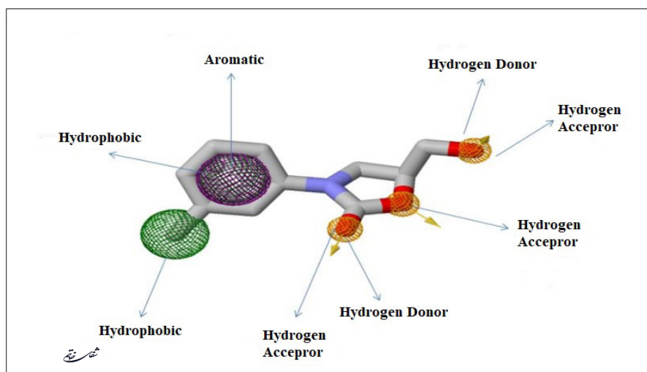
تصویر ۳- تصویر ویژگی‌های فارماکوفوری ترکیب رهبر (تولوکسان) و نمایش ویژگی‌های فارماکوفوری این ترکیب جهت استفاده در جستجوی مجازی توسط سرور zincpharmer جهت یافتن لیگندهای دارای ویژگی‌های فارماکوفوری مشابه آن جهت فرایند داکینگ با آنزیم مونوآمین اکسیداز A-
