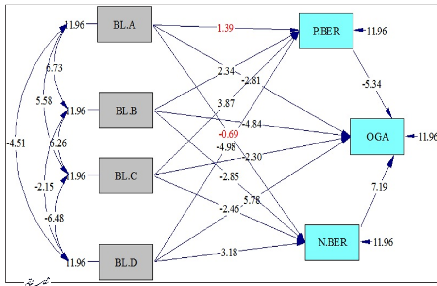
نمودار ۲- آزمون مدل تحقیق (در حالت T-Value)
