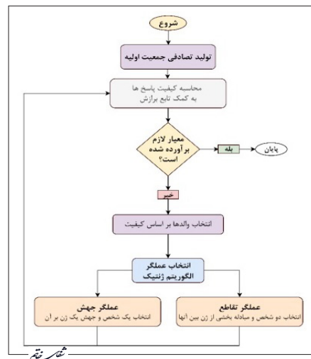
تصویر ۵ - نحوه پیاده سازی الگوریتم ژنتیک
